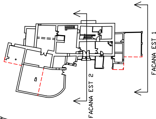
FACANA EST 2
