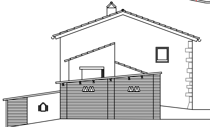
FACANA EST 1
